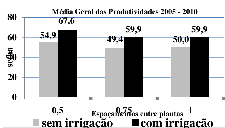
Gráfico 2. Produtividade média após as seis primeiras colheitas entre os espaçamentos entre plantas (0,5; 0,75 e 1,00) com e sem irrigação.
