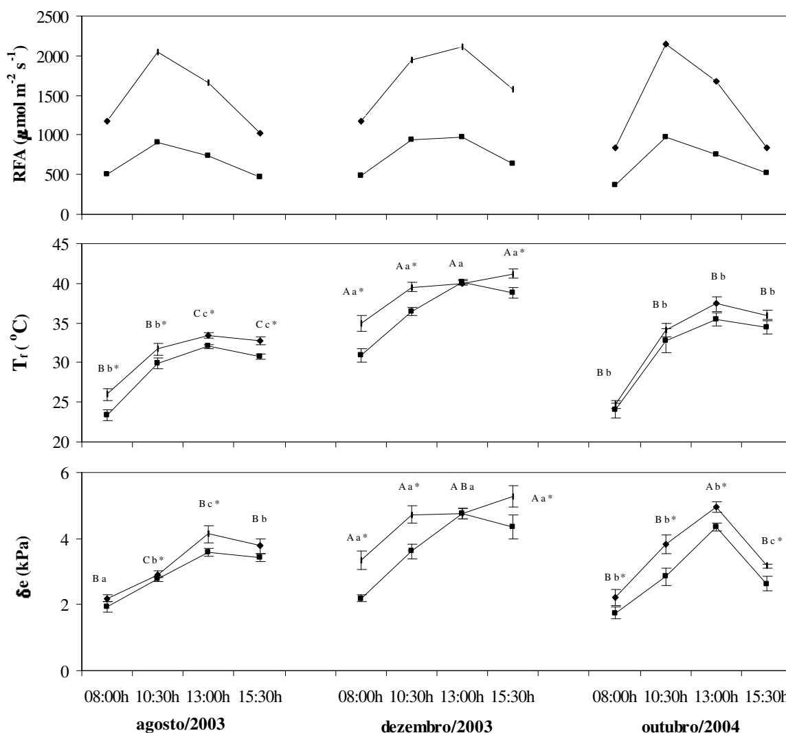
Fig.1 Curso diário da radiação fotossinteticamente ativa (RFA), da temperatura foliar ( T_f ) e do déficit de pressão de vapor entre a folha e a atmosfera ( \delta e ) em plantas de café a pleno sol (linha cheia) e sob sombra (linha tracejada), em três épocas de avaliação. Diferenças estatísticas entre médias obtidas nas três épocas, dentro de um mesmo horário, são indicadas por letras maiúsculas para plantas a pleno sol, e por letras minúsculas, para plantas sob sombra (Newman-Keuls, P = 0,05 ). Asterisco (*) denota diferença significativa (teste t , P = 0,05 ) entre as médias dos regimes de luz, dentro de um mesmo horário e época de avaliação. Exceto para RFA, n = 6 \pm erro padrão da média (EP)
