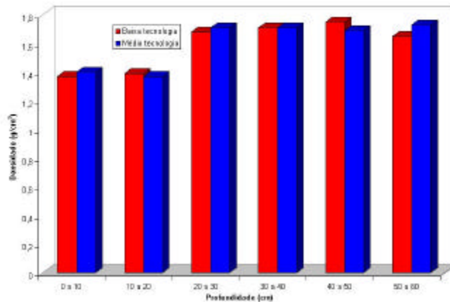
Figura 1 - Valores médios da densidade do solo.
