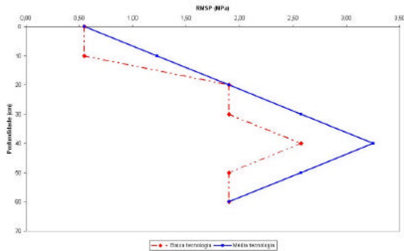
Figura 2 - Valores médios da resistência mecânica do solo à penetração.
